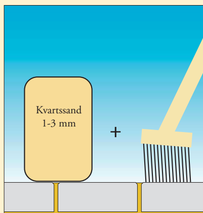
2. Der fejes 2 - 3 gange med skarpt kvartssand, ca. 1 - 3 mm i kornstørrelse. Det er vigtigt, at der ikke er ler eller silt i sandet. Der skal benyttes en stiv kost.
